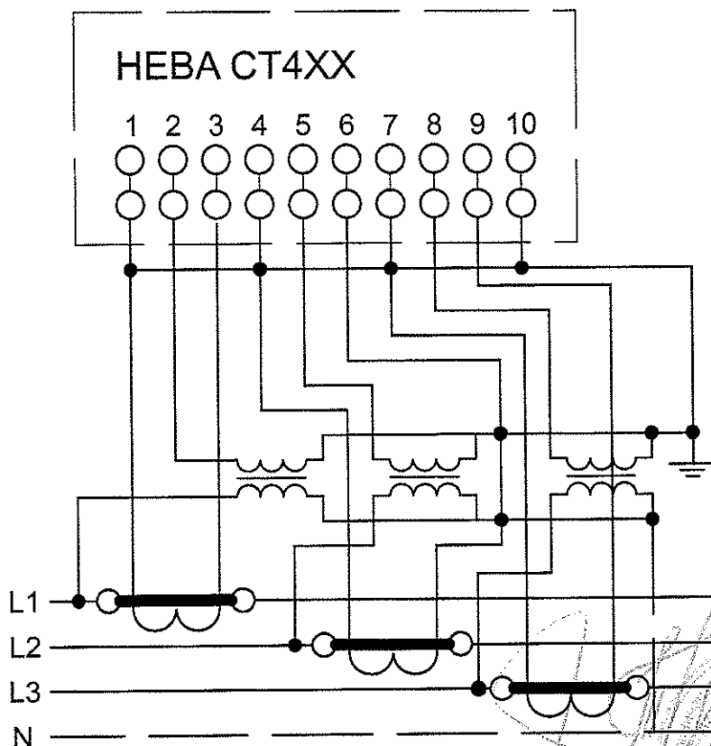
Схема включения счетчика HEBA CT4XX через трансформаторы тока и трансформаторы напряжения в четырехпроводную сеть
