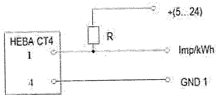
Рисунок 2.1 – Подключение испытательных выходов счетчиков НЕВА СТ4
