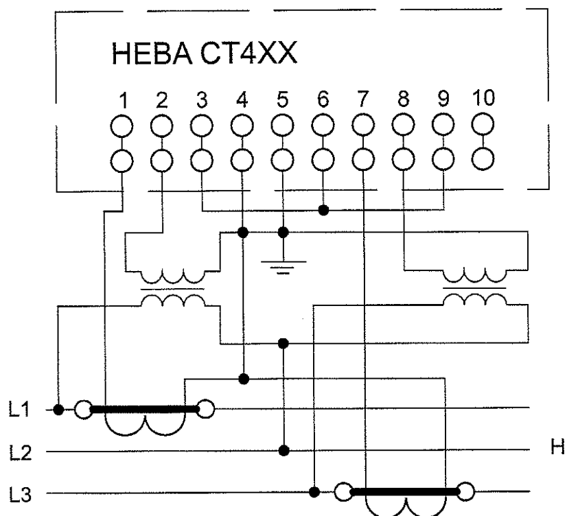
Схема включения счетчика НЕВА СТ4ХХ через трансформаторы тока и трансформаторы напряжения в трехпроводную сеть
