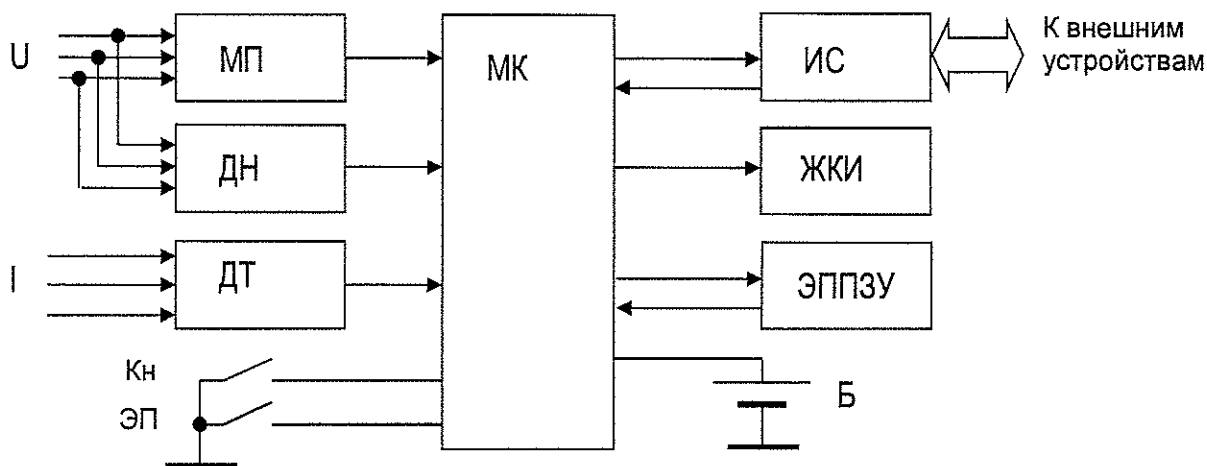
Рисунок 1.2 – Функциональная схема счетчика.
