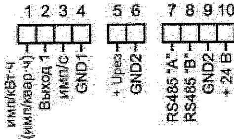
Схема подключения НЕВА СТ4ХХ без дополнительного модуля входов/выходов
