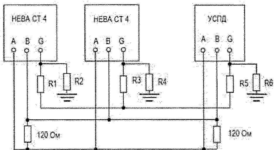
Рисунок 2.2 – Схема подключения счетчиков к интерфейсной линии EIA 485
