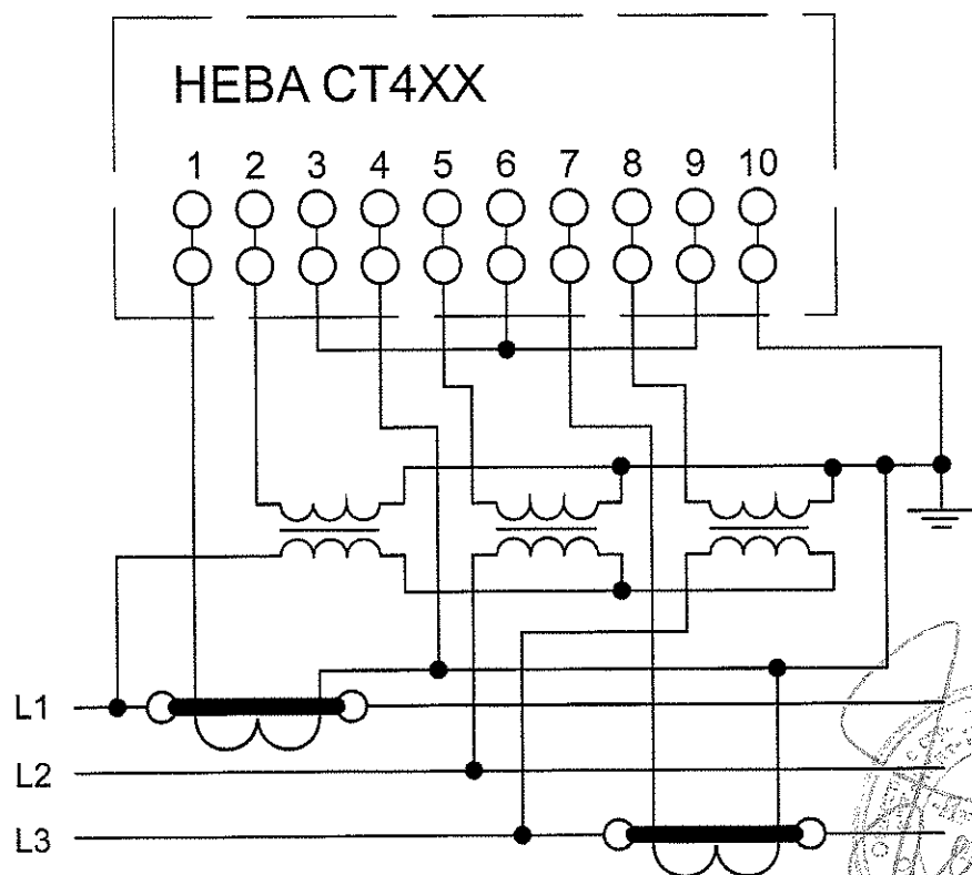
Схема включения счетчика НЕВА СТ4ХХ через два трансформатора тока и три трансформатора напряжения в трехпроводную сеть
